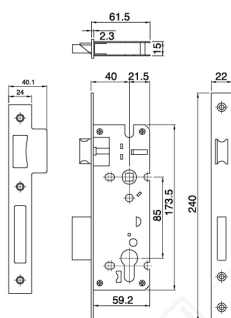
MTS IL DL840 AL F/AL PROFILE SSS
