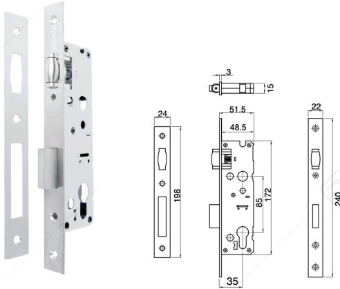
MTS RL DL83585 SSS
