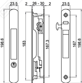
KS RA6 NA Available : • WH • BK • YB1C
