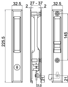
KS J5K ONE SIDE KEY BK Available : • NA • WH • BA
