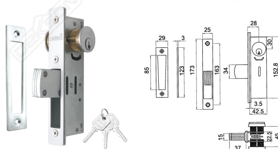
KC 8128 (PJ) Available: KC 8128 (PD)
